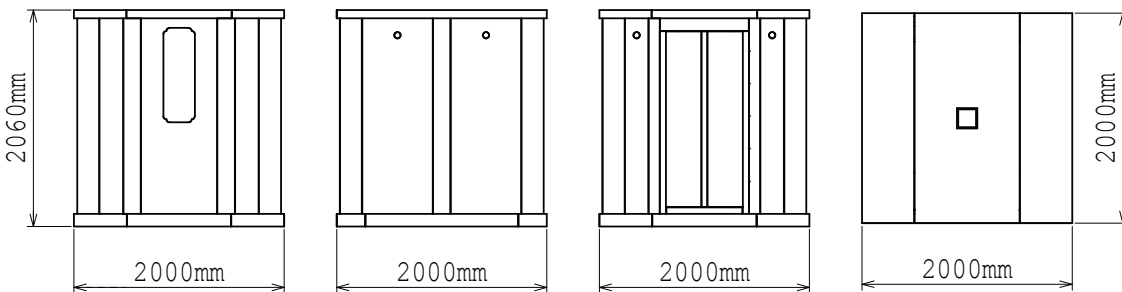
[正面図]
