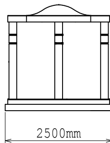
[背面図]
