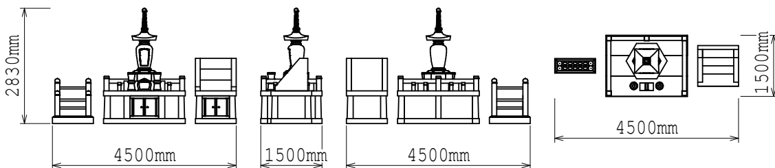
[正面図]
