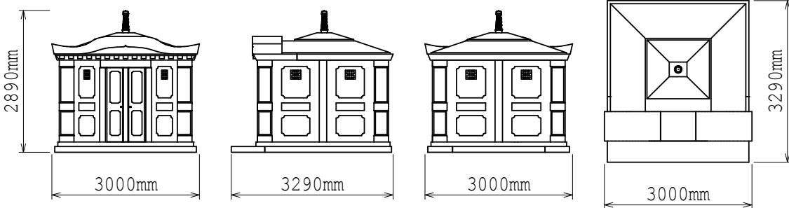
[正面図]
