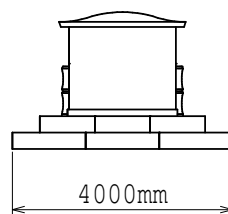
〔背面図〕
