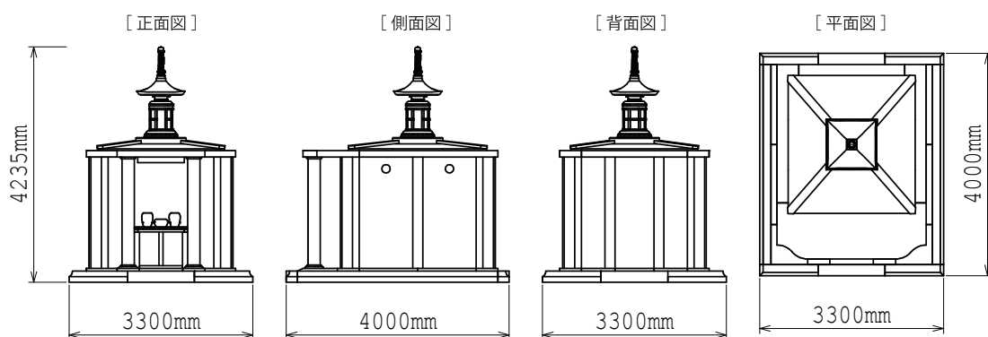
外形寸法図
